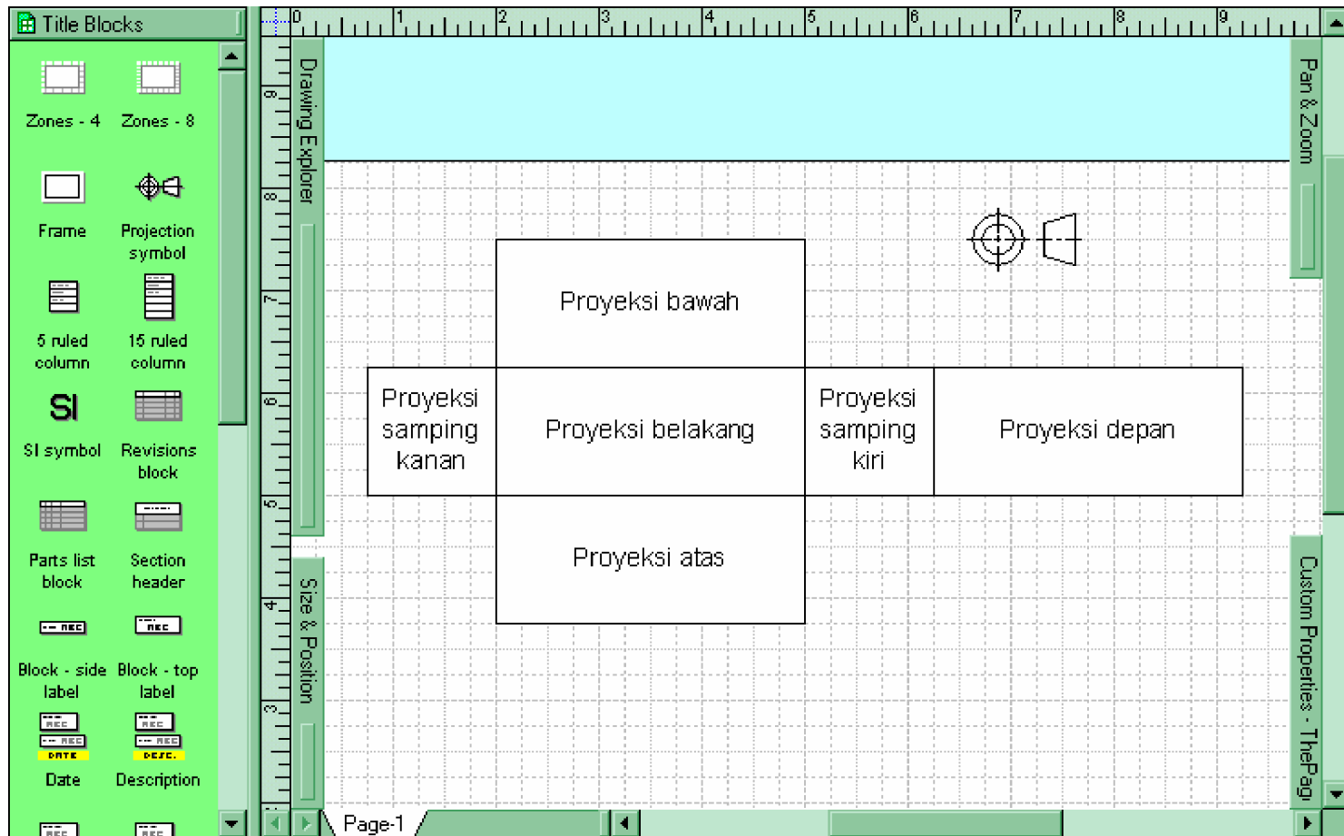
Gambar 23. Bukaan Balok Hasil Proyeksi Sudut Ketiga
