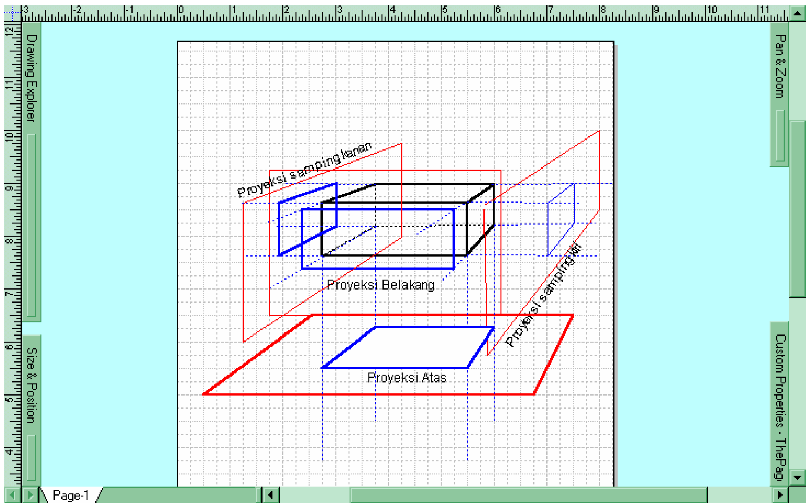
Gambar 21. Hasil Proyeksi Sudut Ketiga/ Cara A.
